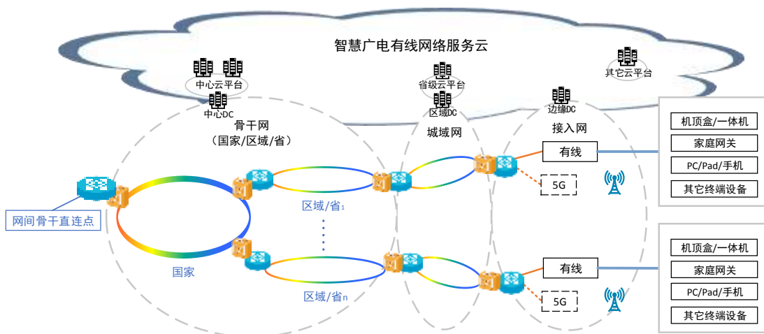
图 1 有线电视网络技术架构示意图
